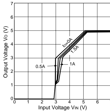
Rise Characteristics(SI-3050C)
