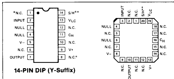
SMP-11BRC/883 LCC PACKAGE (RC-Suffix)
