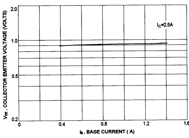
V_{BE(SAT)} - I_B
