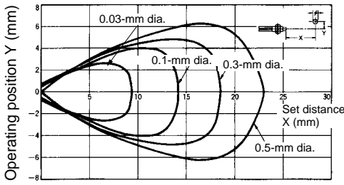
E32-CC200 with E3X-NT11
