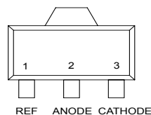
M1 Package (SOT-89)
