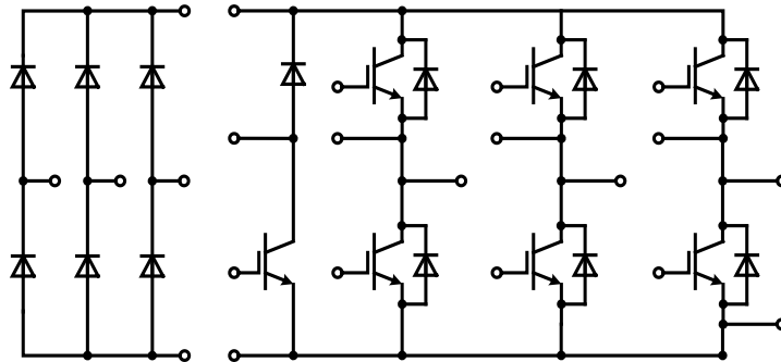
Rectifier
