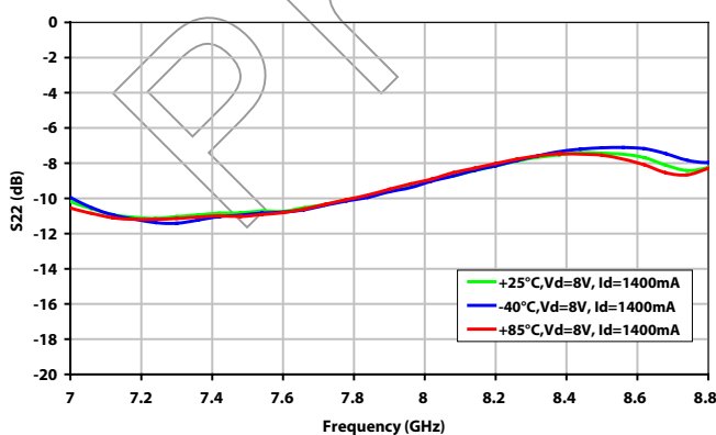
XP1050-QJ: S22 Vd=8V, Idtot=1400mA
