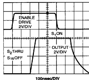
Figure 7. Enable Delay ( t_{ON(EN)} , t_{OFF(EN)} )
