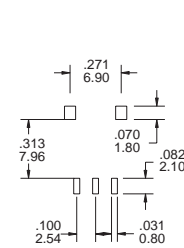
ES-27A
