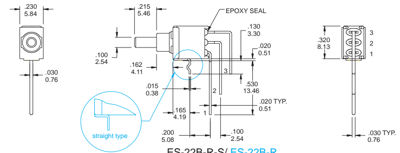
ES-22B-R-S/ ES-22B-R
