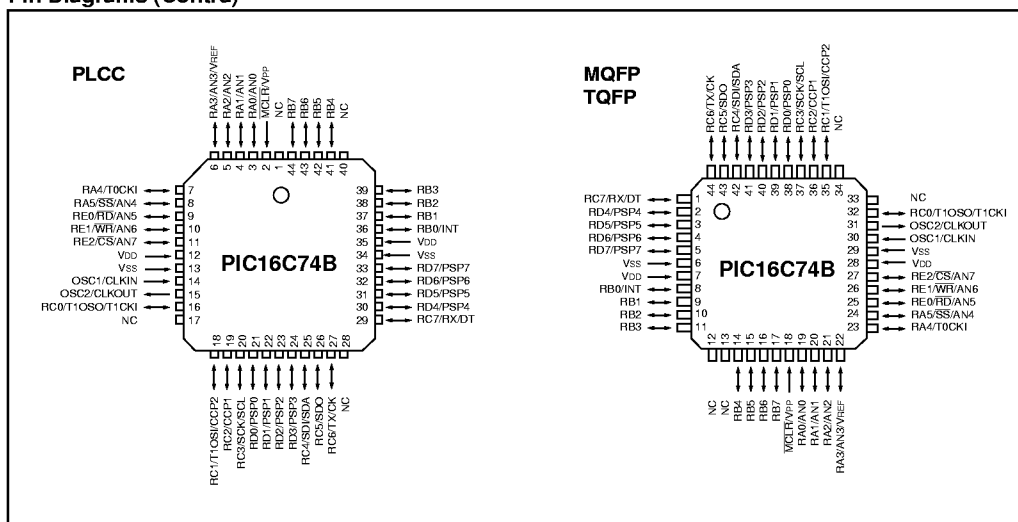
Pin Diagrams (Cont'd)
