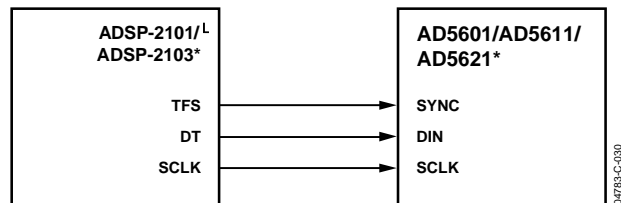
Figure 29. AD5601/AD5611/AD5621 to ADSP-2101/ADSP-2103 Interface
