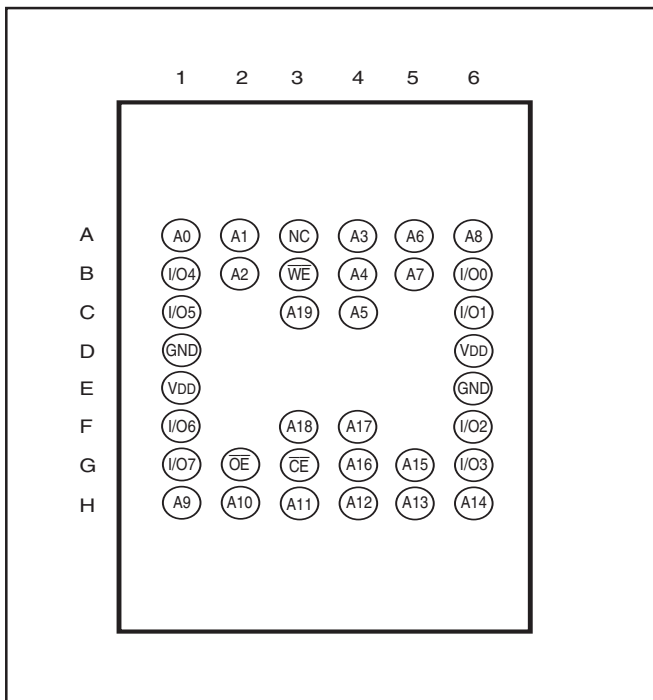
36 mini BGA (B) (9mm x 11mm)
