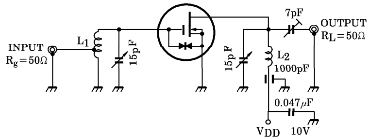
Fig. 1 G_{ps} , NF TEST CIRCUIT
