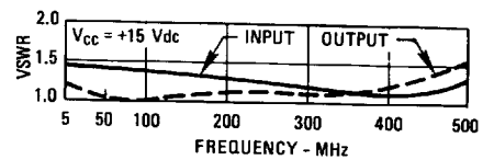
VSWR
