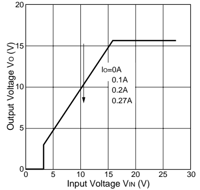
Output Voltage(SI-3157B)
