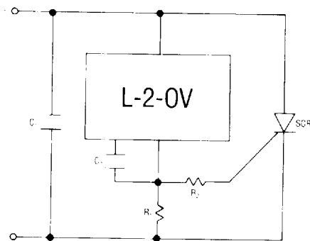
(5, 12, 15 VOLT MODELS)
