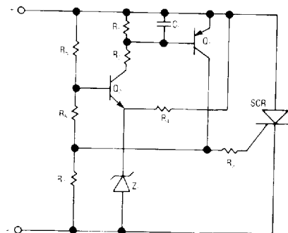
(24, 30 VOLT MODELS)
