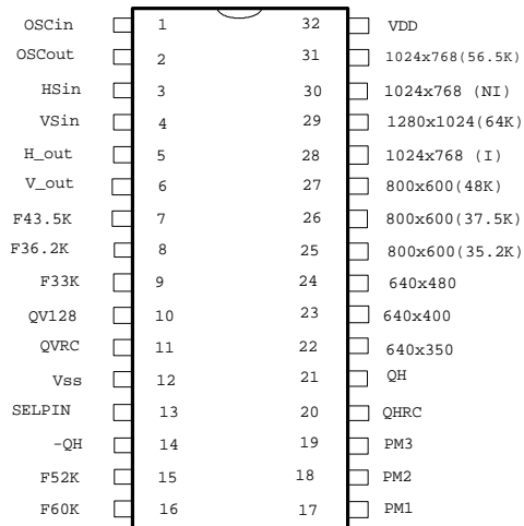
WT8045N32
