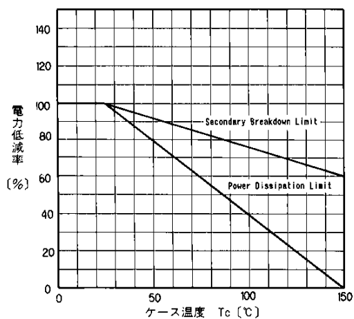
ASO低減特性 ASO Dersting
