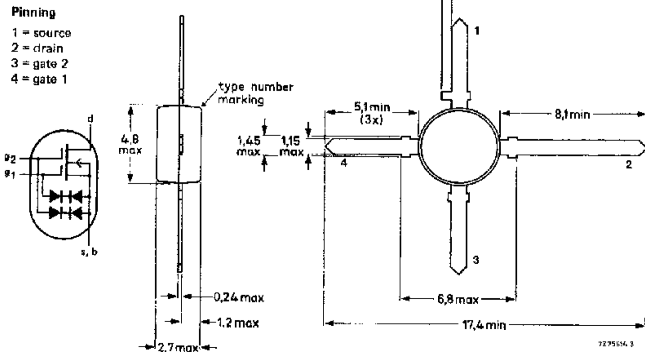
Fig.1 SOT103.
