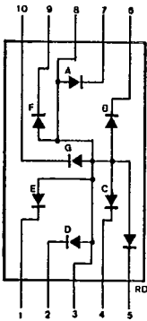
A. LTS-6x60
