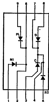
D. LTS-6x95
