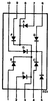
B. LTS-6x80
