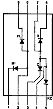
C. LTS-6x75
