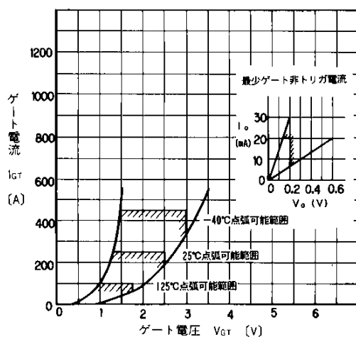
ゲート特性 Gate Characteristics
