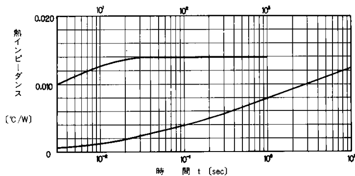
過渡熱インピーダンス
