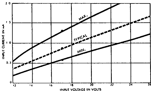
Dwg. No. A-10,225A
