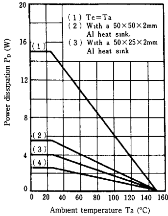
P_D - T_a (PU3213)
