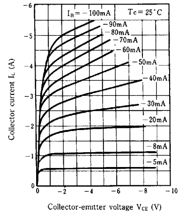
I_C - V_{CE}
