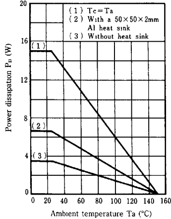
P_D - T_a (PU4213, PU4513)
