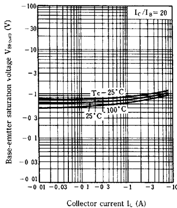
V_{BE(sat)} - I_C
