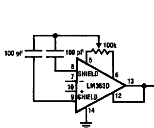
d. AC CMRR
