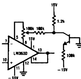
e. Negative PSRR
