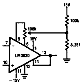
f. Positive PSRR
