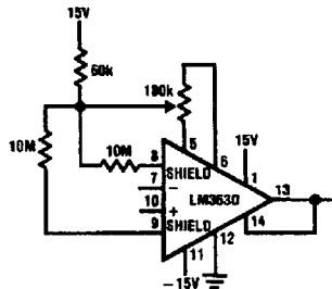
c. DC CMRR
