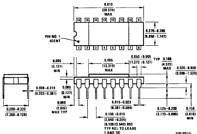
Hermetic Dual-In-Line Package (D) Order Number LM363D NS Package Number D16C
