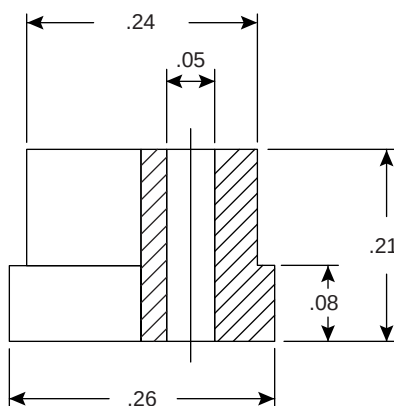
351-1200 Bezel Base
