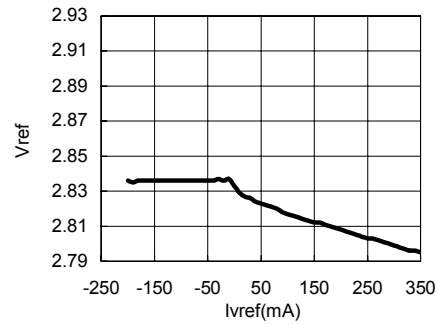
Vref - Ivref@Vtpwr=5V;T=24°C
