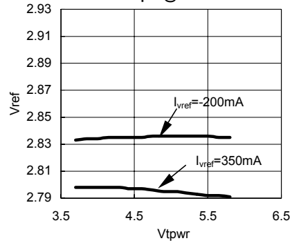
Vref - Vtpwr@T=24°C
