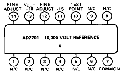
Device Type -3, -4
