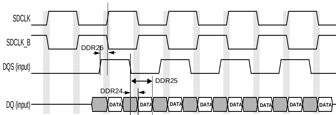
Figure 36. DDR2 SDRAM DQ versus DQS and SDCLK Read Cycle
