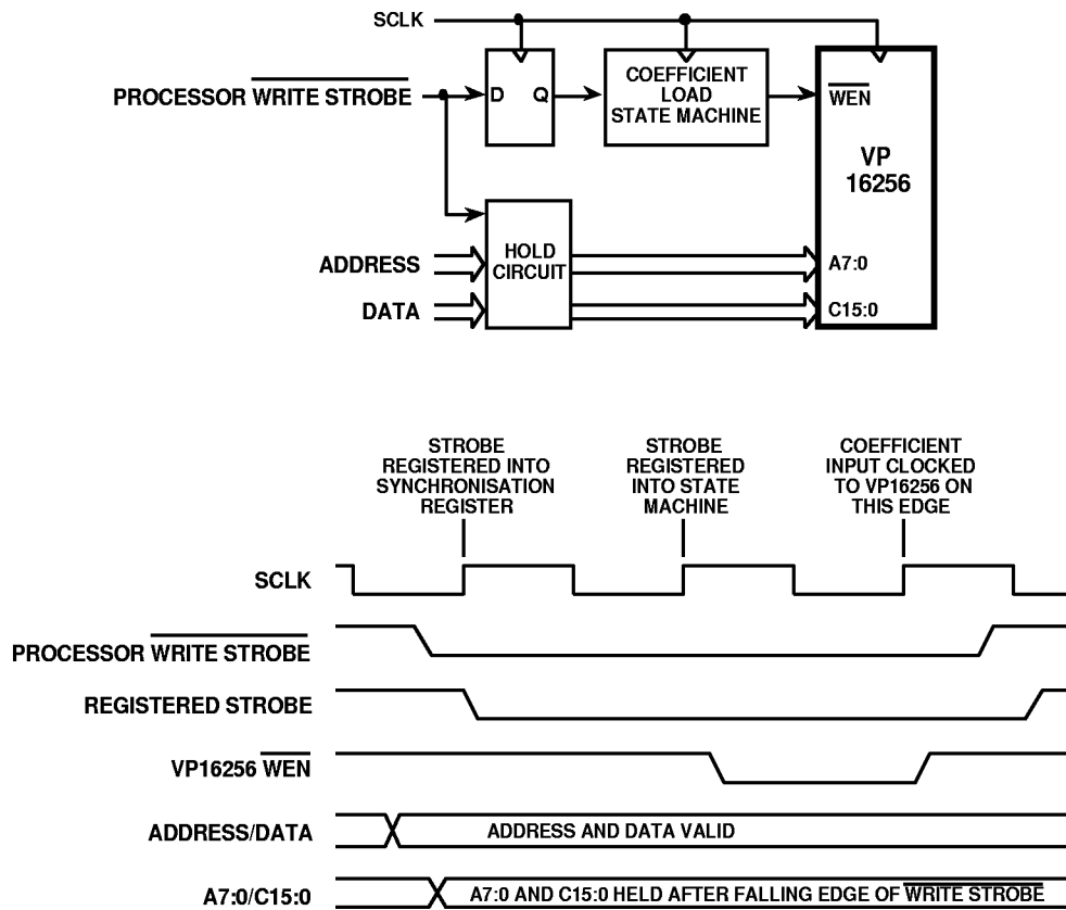
Fig. 17 Remote Master synchronisation
