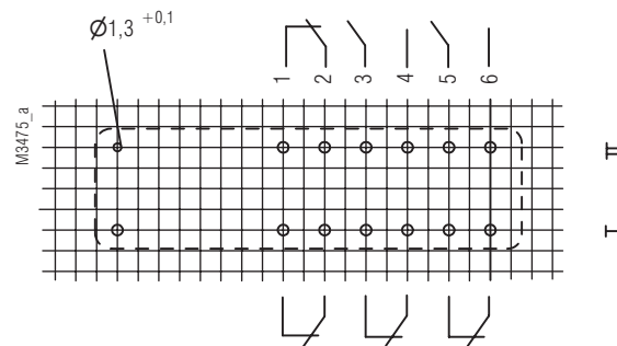
Connexions des picots OA 5612.18/...L1 3NO / 3NF
