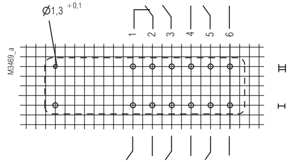
Connexions des picots OA 5612.54/...L4 2NF / 4NO
