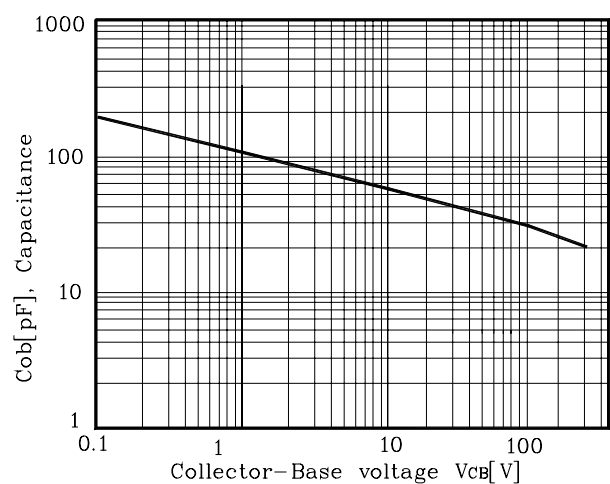
Fig. 6 Capacitance
