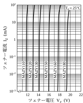
I_Z - V_Z
