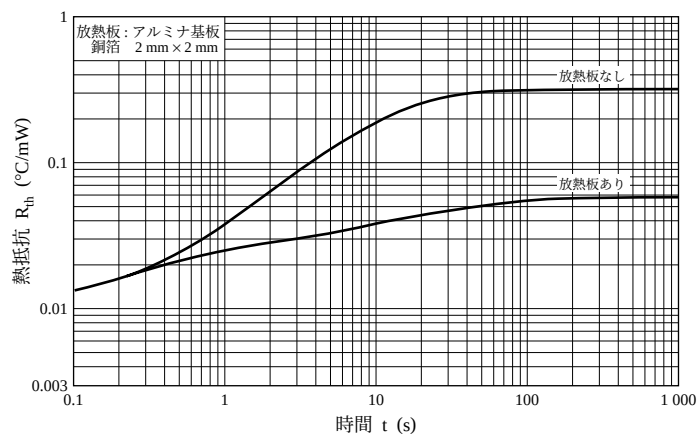
R_{\text{th}} - t
