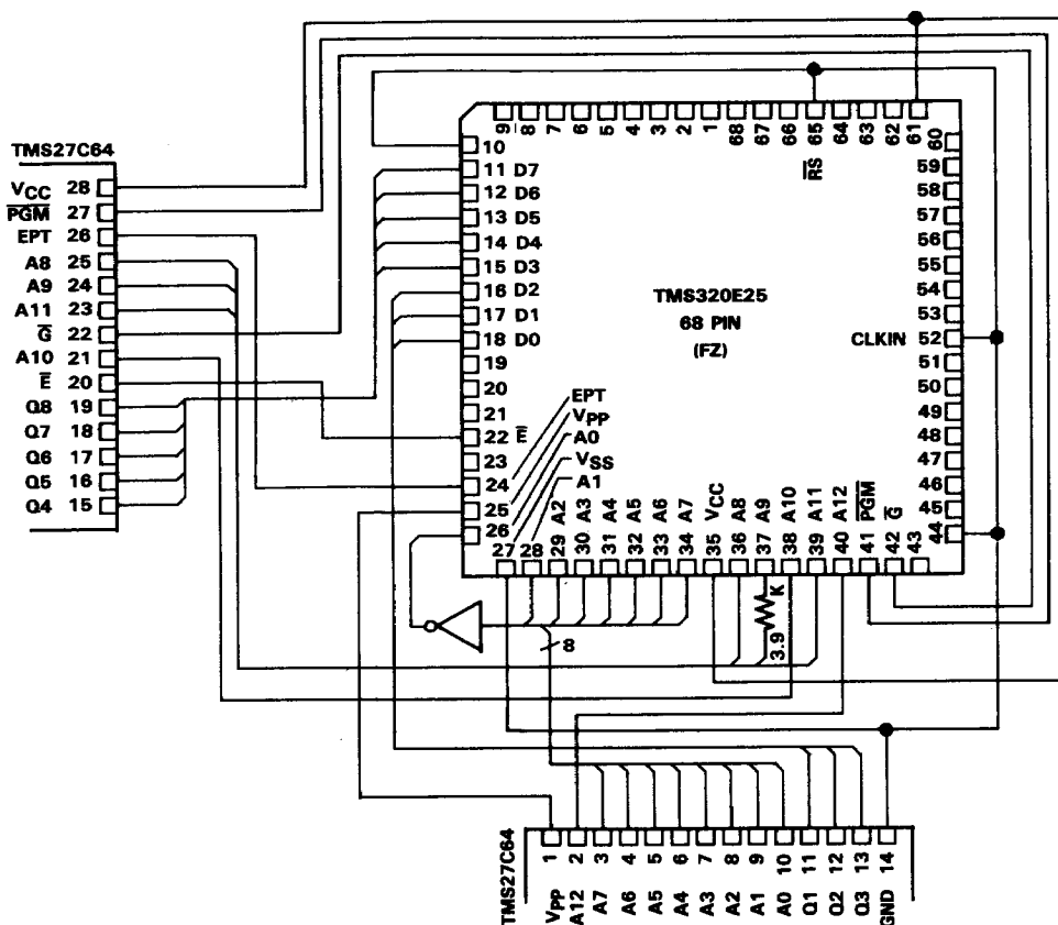
PIN NOMENCLATURE (TMS320E25)
