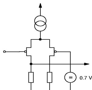
Fig. 3-14: Input Pin 30
