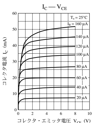
Tr2 部特性図
