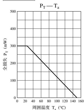
共通特性図
