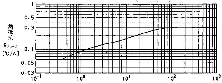
時間 t (sec) 過渡熱抵抗(ダイオード)特性 Transient Thermal Resistance (F.R.D)
