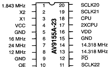
20-Pin DIP or SOIC K-4, K-7
