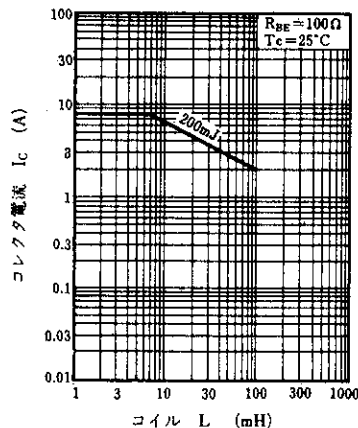
誘導負荷特性
