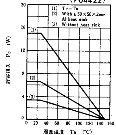
P_D - T_a (PU4122, PU4422)
