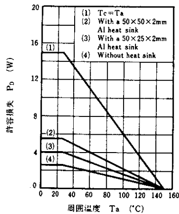
P_D - T_a (PU3122)
