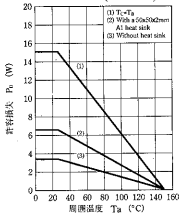
P_D - T_a (PU4137, PU4437)
