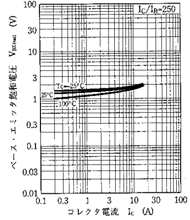
V_{BE(sat)} - I_C
