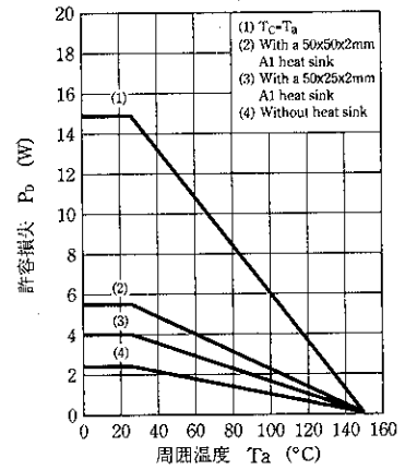
P_D - T_a (PU3137)
