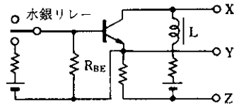
*E s /b試験回路(1回路)
