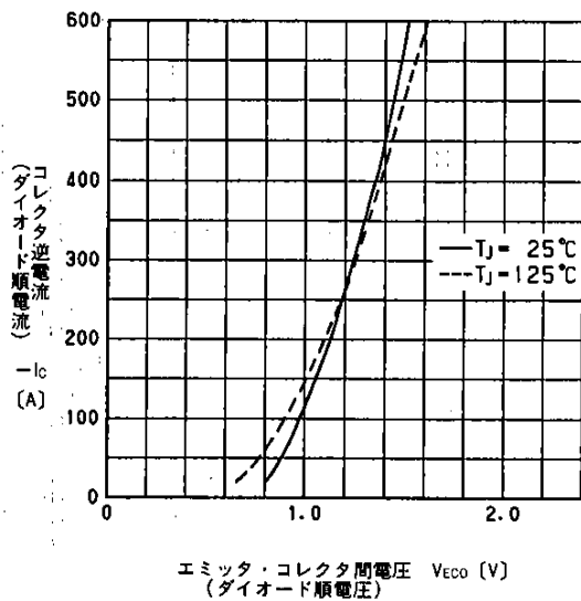
高速フリーホイーリングダイオード順電圧特性 Forward Voltage of Free Wheeling Diode
