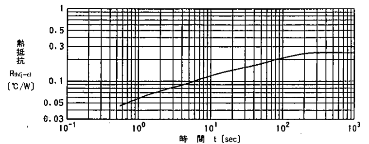
過渡熱抵抗(ダイオード)特性 Transient Thermal Resistance (F.R.D)
