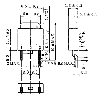
2SA1412-Z 外形図
