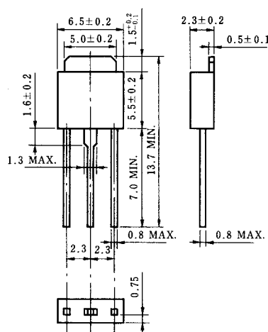
2SA1412外形図
