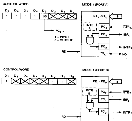
Figure 11 : MODE 1 INPUT
