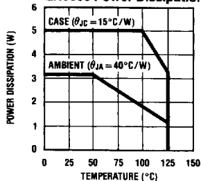
LH0063 Power Dissipation
