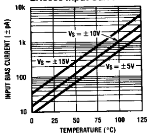
LH0063 Input Current
