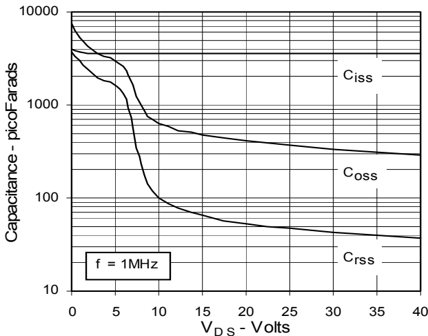
Fig. 11. Capacitance
