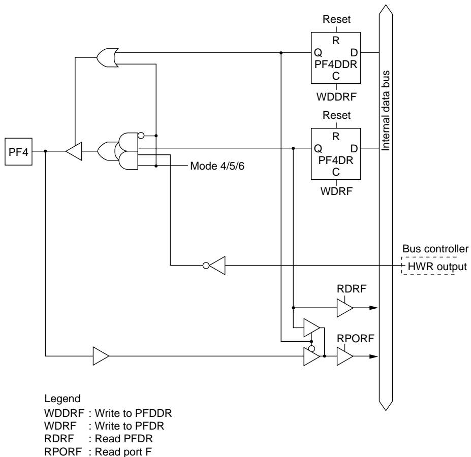
Figure C-12 (d) Port F Block Diagram (Pin PF4)
