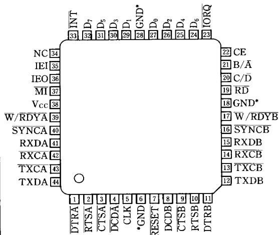
LH0087M/LH0087AM
