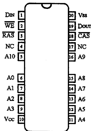
20 (26) SOJ
