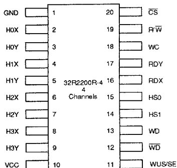
20-Lead SOV, SOL
