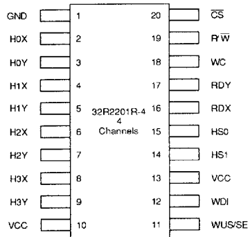
20-Lead SOV, SOL
