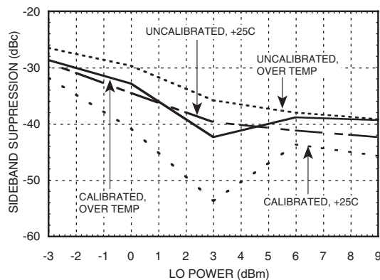
Sideband Suppression* vs. LO Power@ 5200 MHz
