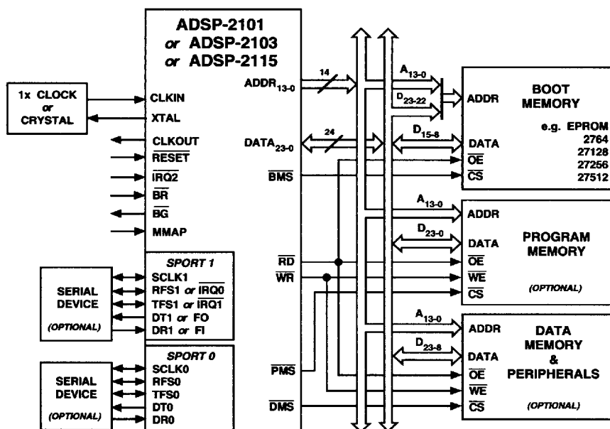
Figure 3. ADSP-2101/ADSP-2103/ADSP-2115 System
