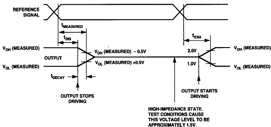
Figure 27. Output Enable/Disable
